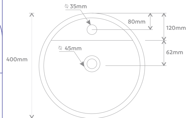
Vista Superior
