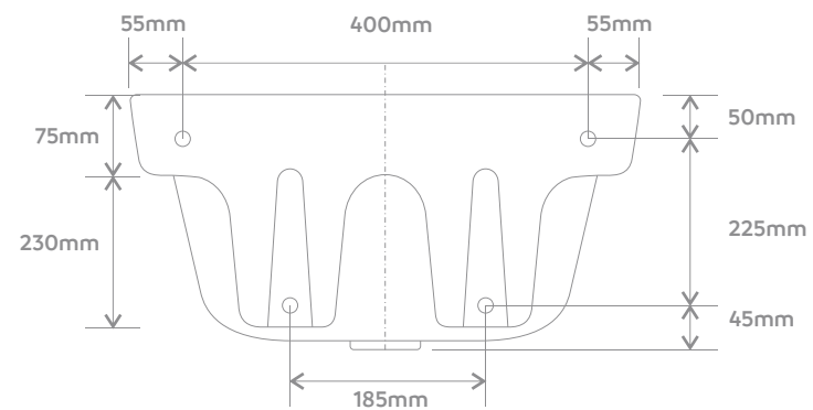
Vista Posterior
