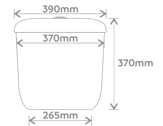
Vista Lateral
